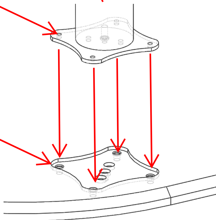
Винт М6*12
